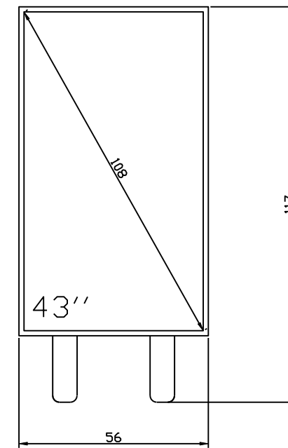
Prospetto laterale
